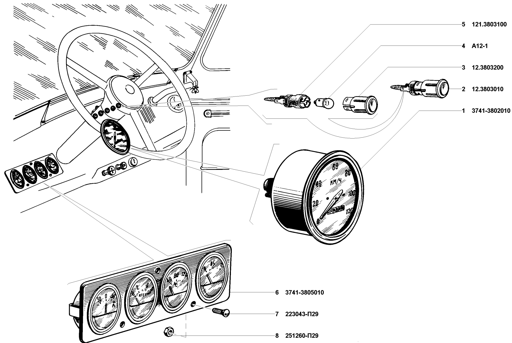
Рис. 136. Спидометр (3802), фонари контрольных ламп (3803) и щиток приборов (3805)
